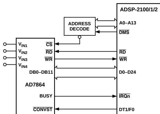
Figure 20. AD7864–ADSP-2100 Interface
