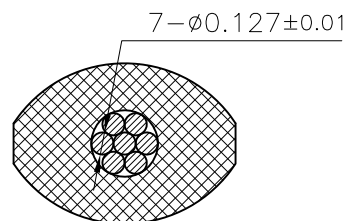
SECTION A-A (4:1)
