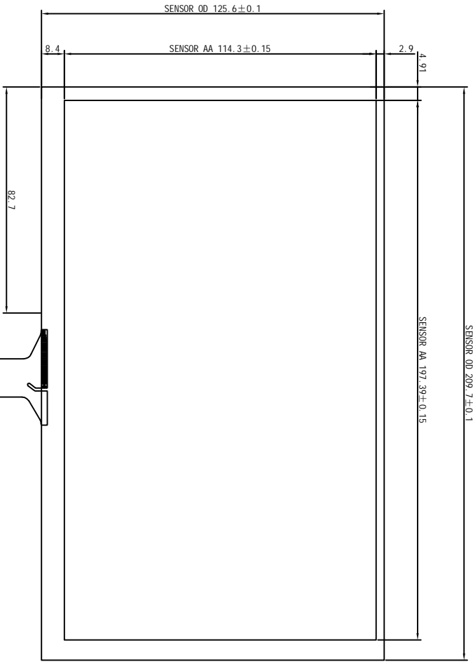
正视图
